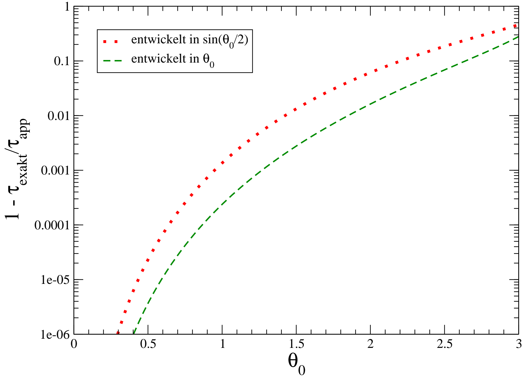
Periode des mathematischen Pendels: Vergleich der Approximationen
