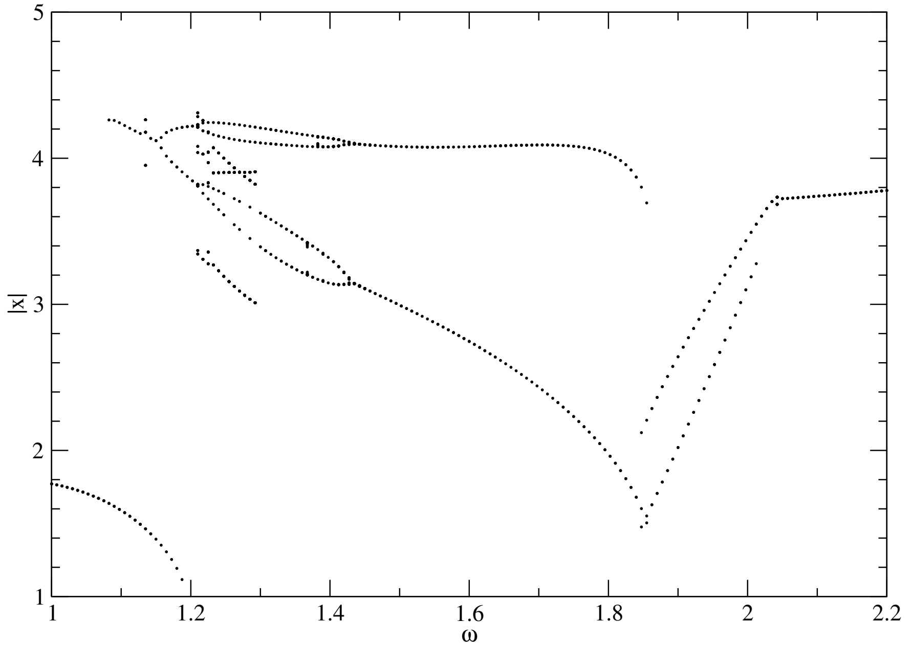
Poincare Verschiebung bei \cos(\omega t) = -1 : f = 20 , \gamma = 0.1
