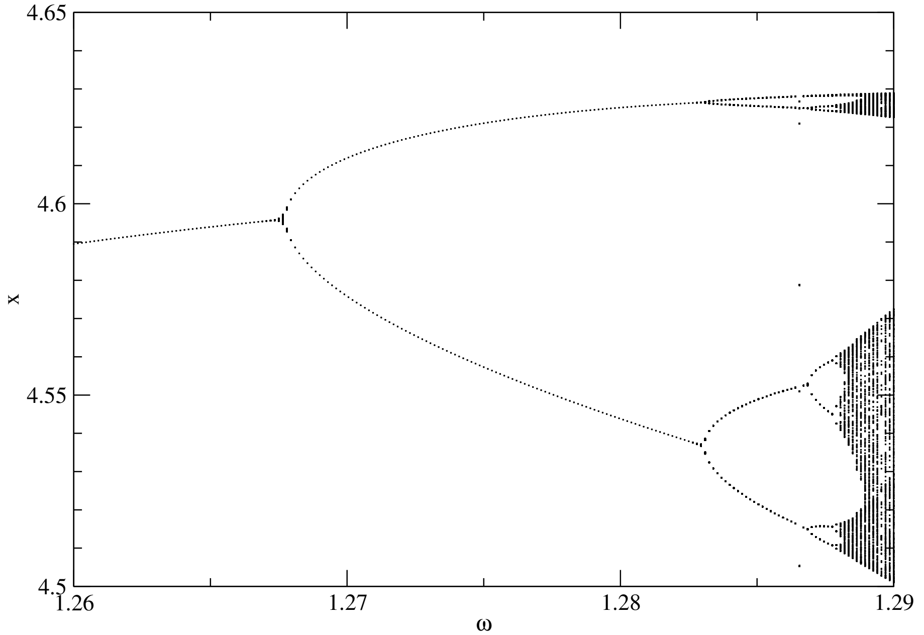
Poincare Verschiebung bei \cos(\omega t) = 1 : f = 25 , \gamma = 0.1
